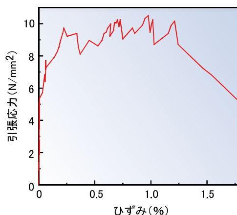
一軸直接引張試験による応力ひずみ関係
