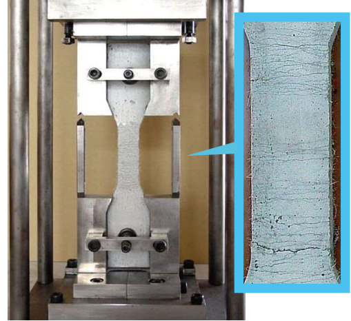
ダンベル型一軸直接引張試験による性能評価 引張終局ひずみ：平均値4.76%（規格値0.5%以上）
